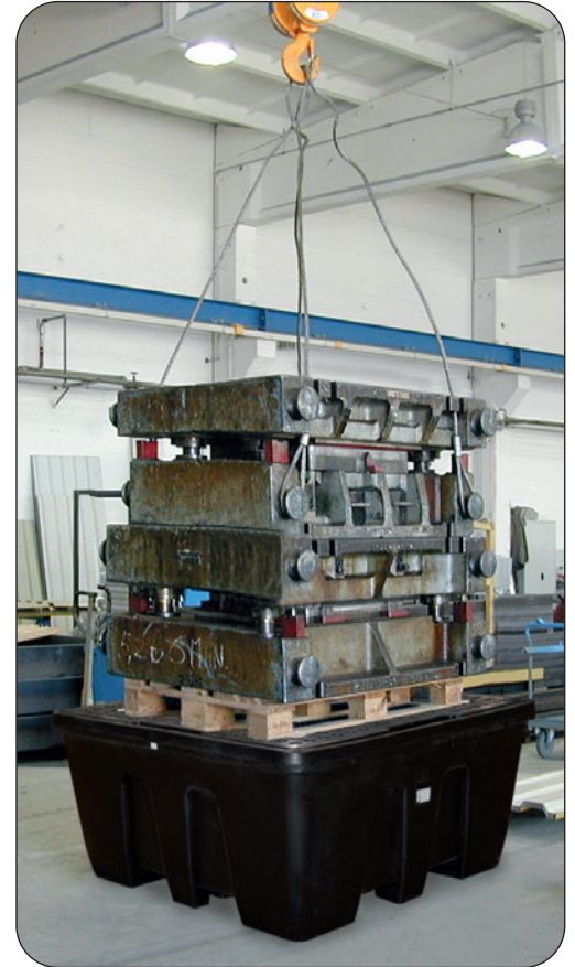
Auffangwanne PE-KT-15 unter einer Prüflast von 8.000 kg
