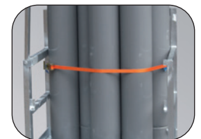
Zurrgurt für alle Typen, als Zubehör erhältlich, Länge 3 mtr., Artikel-Nr. Z50-1921-A
